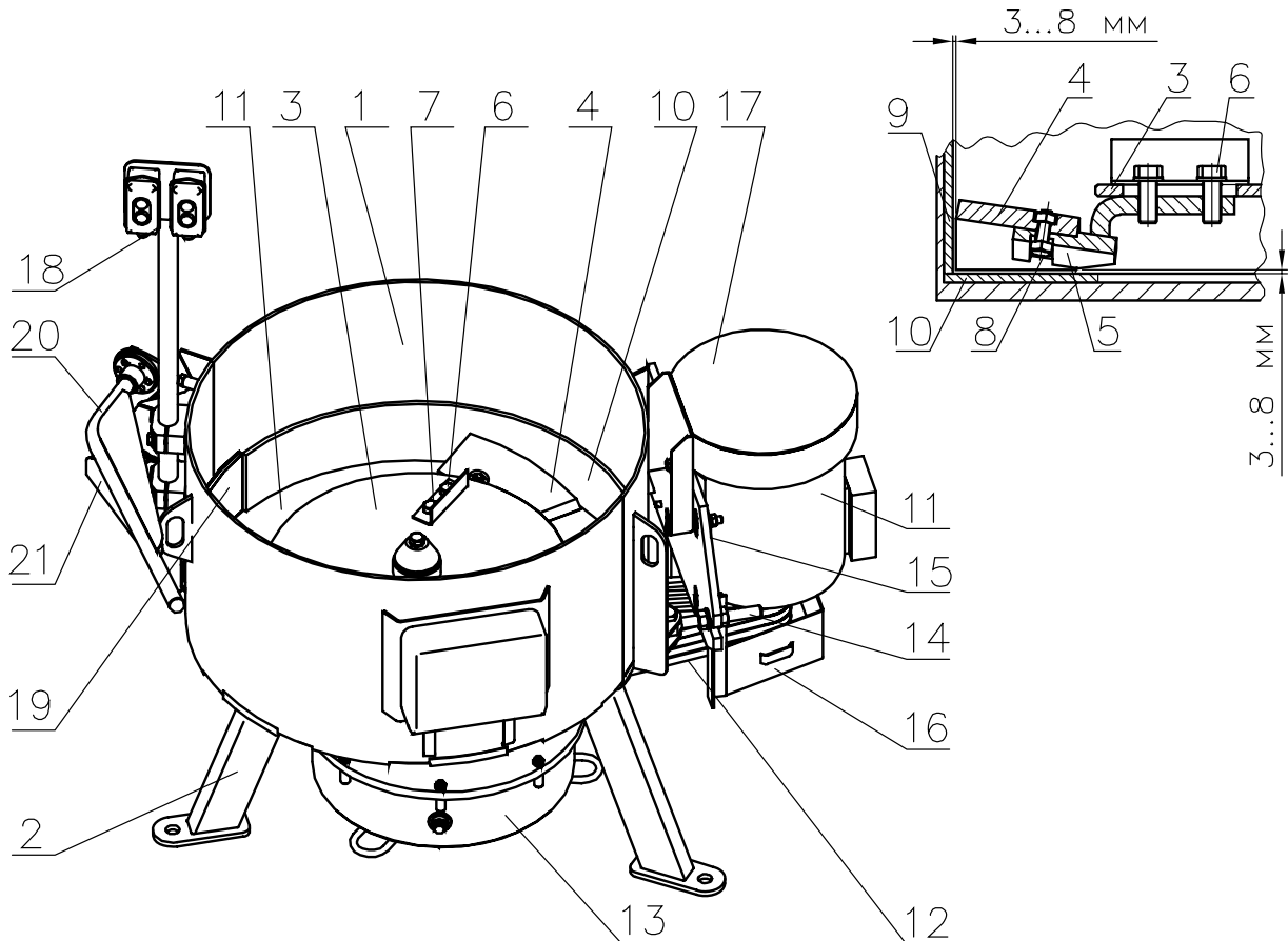
Рис. 8. Смеситель.
