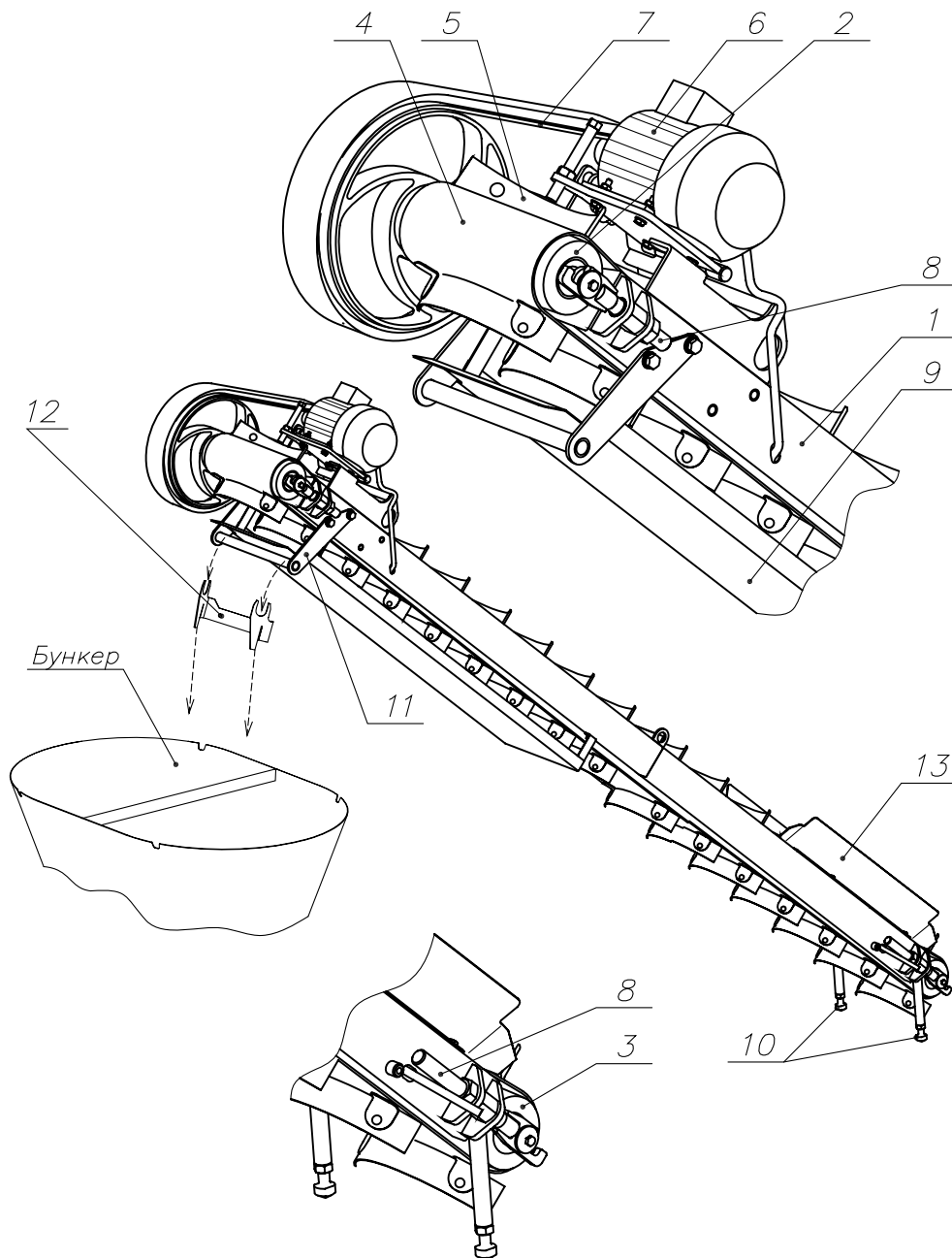
Рис. 10. Транспортер
