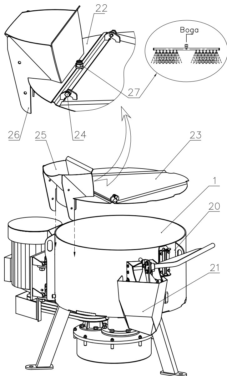
Рис. 8а. Крышка смесителя.
