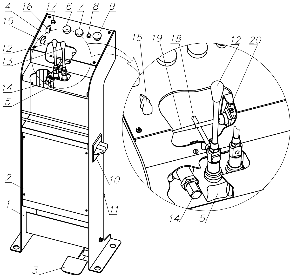
Рис. 3 Пульт управления.
