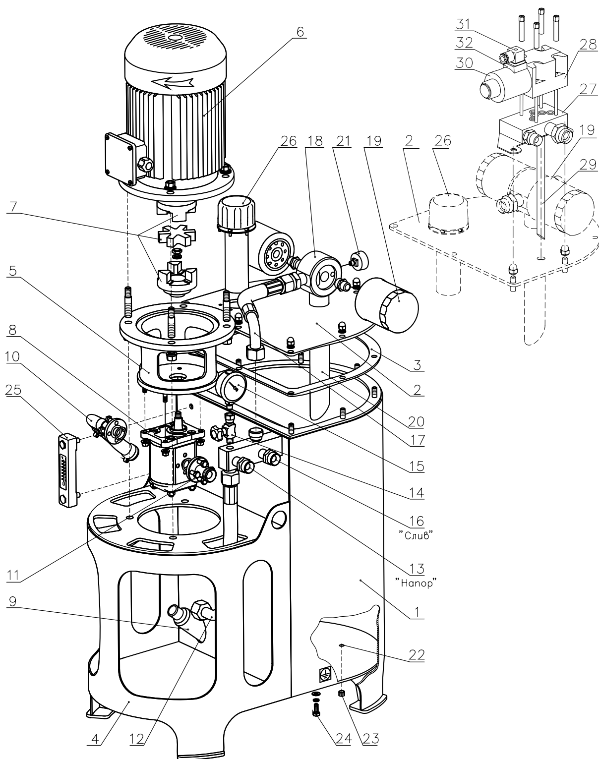
Рис. 5. Установка насосная.
