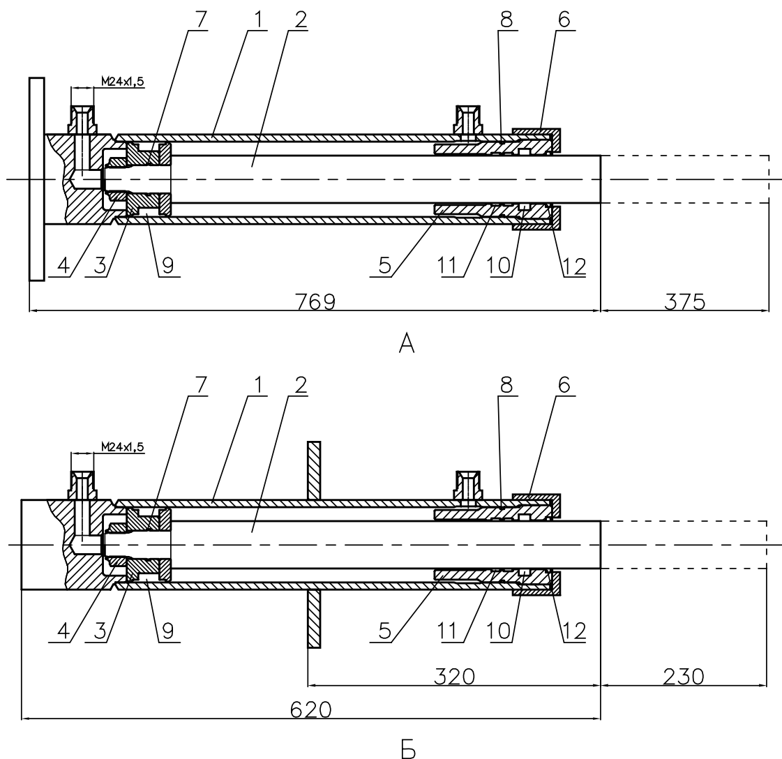
Рис. 7. Гидроцилиндры.
