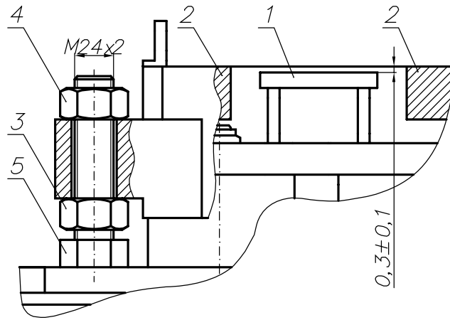
Рис. 20. Схема настройки зазора.
